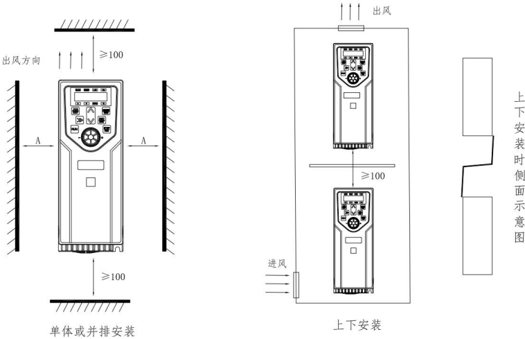
图 3.2-1 变频器安装示意图
