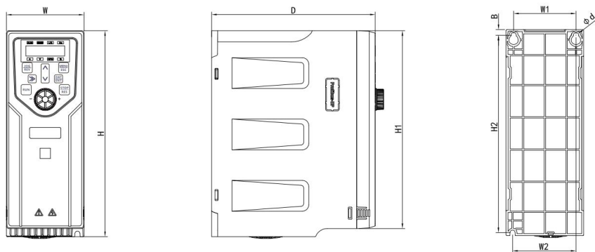
图 2.4-1 FG270-4T (1.5kW~5.5kW) 产品外形及安装尺寸示意图
