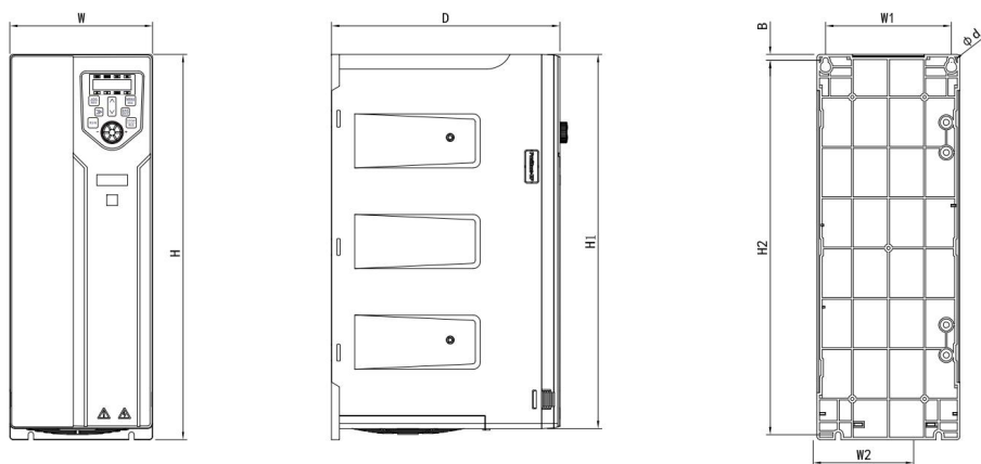
图 2.4-2 FG270-4T (7.5kW~30kW) 产品外形及安装尺寸示意图
