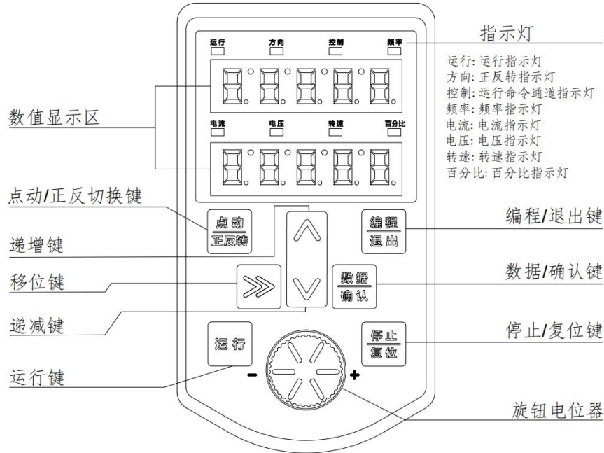
图 4.1-1 操作面板示意图
