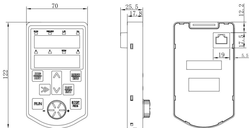
图 2.5-1 LED 键盘外形尺寸
