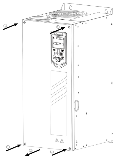
图 3.3-3 钣金外壳盖板的拆卸和安装示意图
