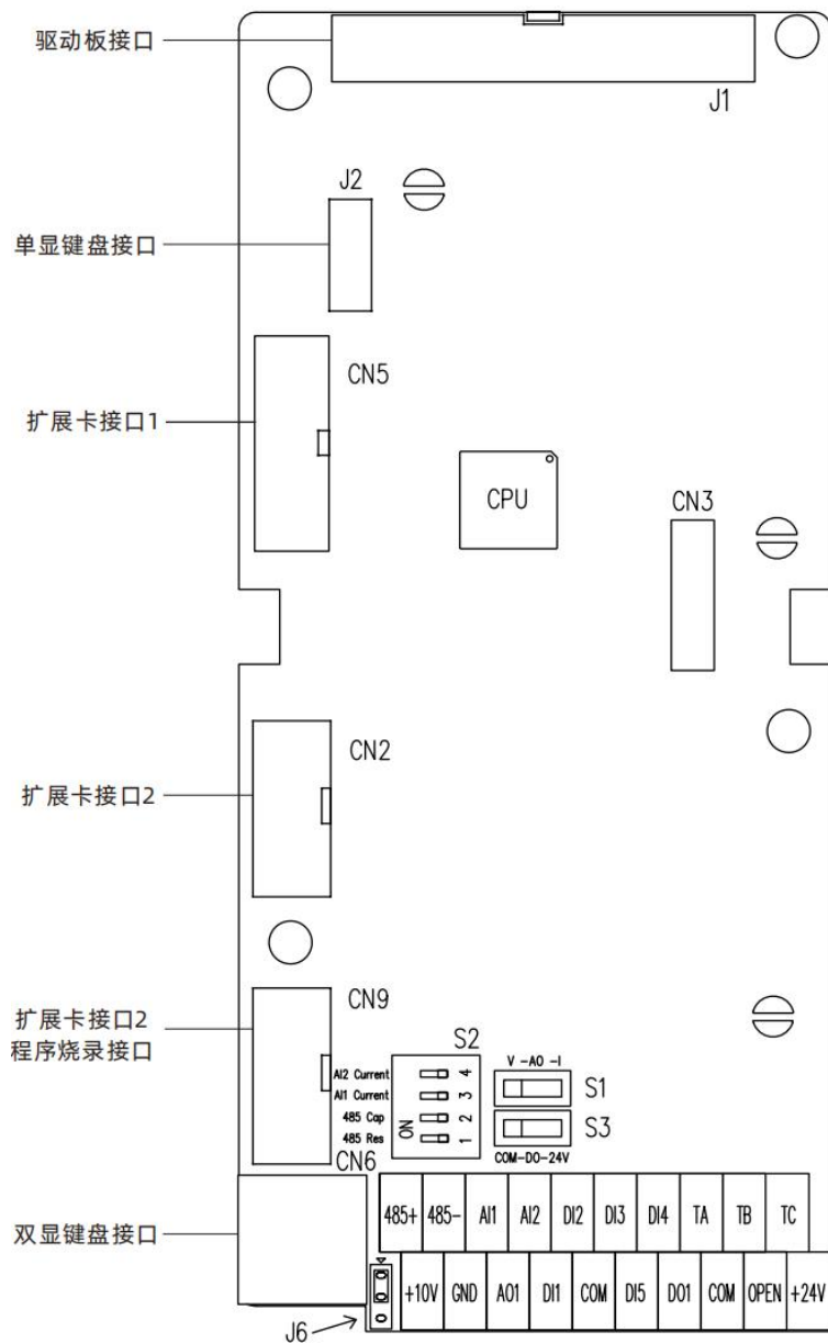
图 3.5-1 控制板布局示意图
