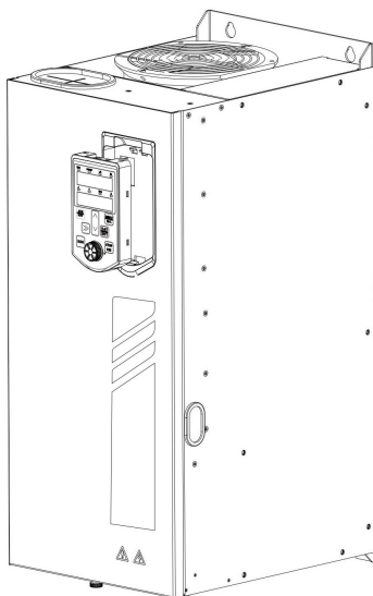
图 3.3-1 操作面板的拆卸和安装示意图
