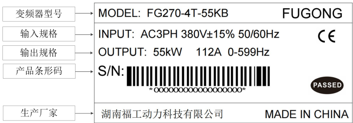
图 2.2-1 铭牌说明
