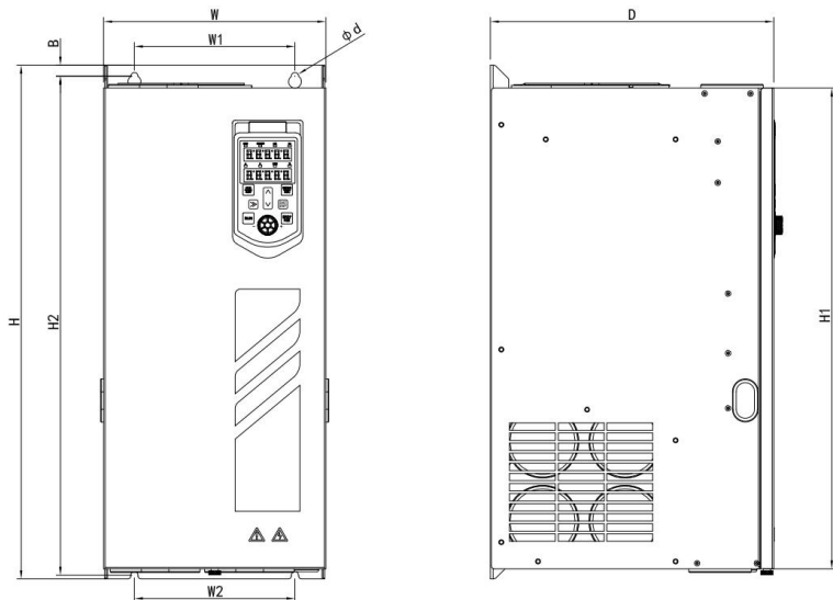
图 2.4-3 FG270-4T (37kW~400kW) 产品外形及安装尺寸示意图
