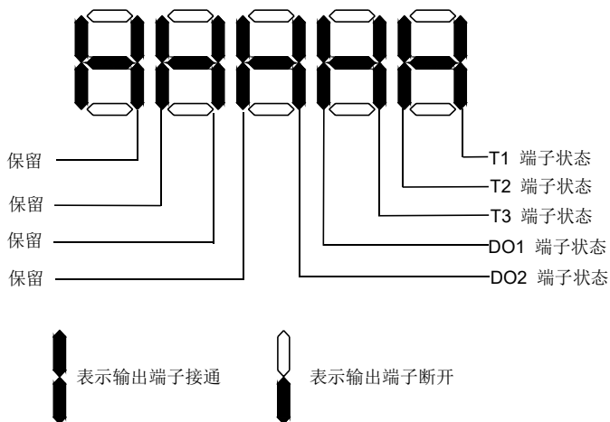
图 5.5-2 输出端子接通/断开状态示意图
