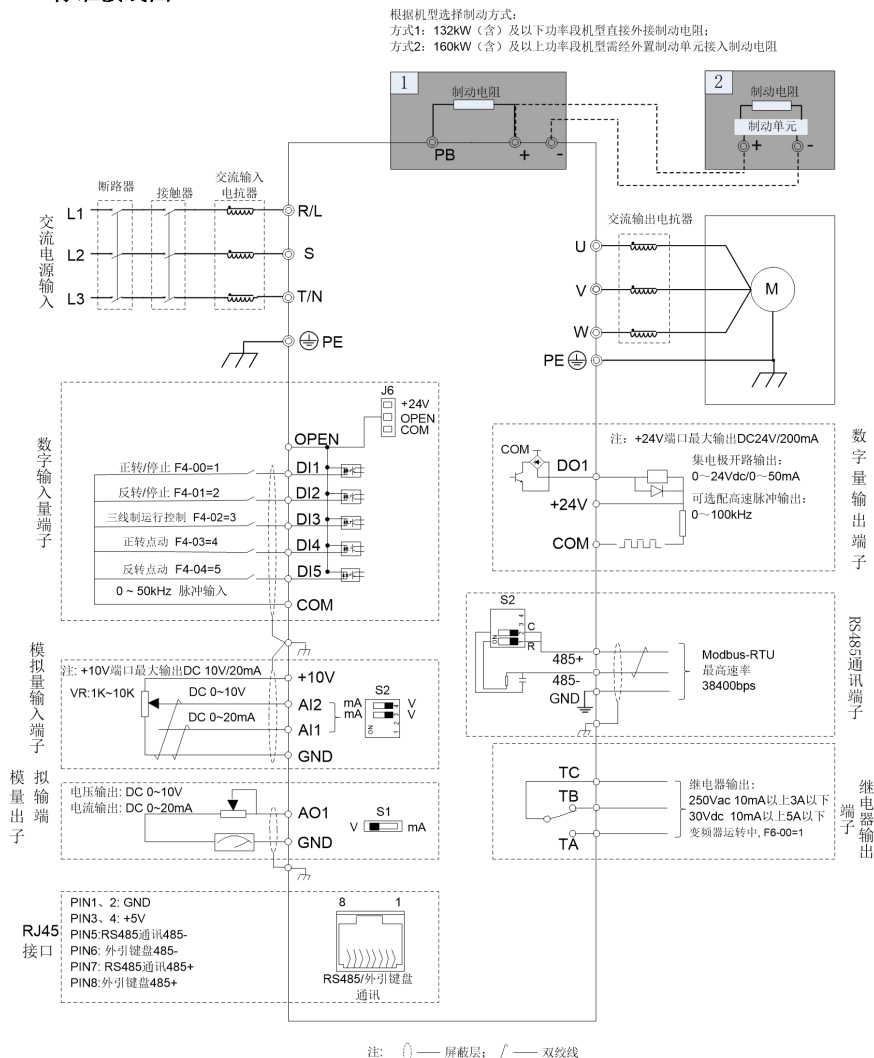
图 3.5-1 变频器标准接线示意图
